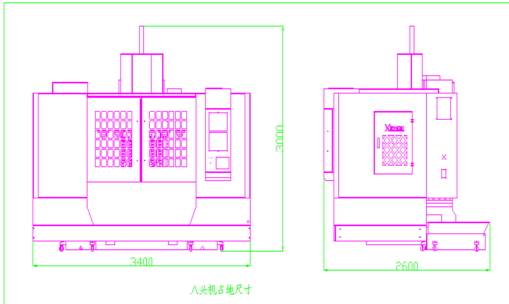
DK850-8 外型尺寸图、吊装示意图:
