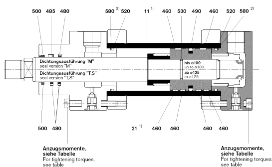
Anzugsmomente Rundzylinder/ torques for mill-type cylinders CDH1 / CDH2 / CDH3 Dichtungsausführung M, T, S Seal versions M/T/S
