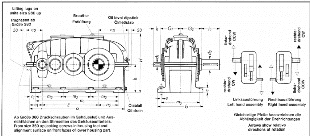
Maße, Gewichte und Ölmengen Dimensions, weights and oil quantities
